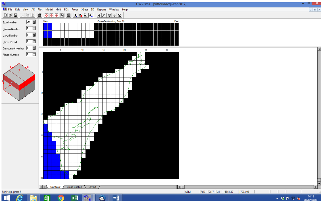
Figura 4.5 Delimitazione dell'area dell'acquifero superficiale individuato nella piana di Vittoria in cui è stato applicato il modello MODFLOW
