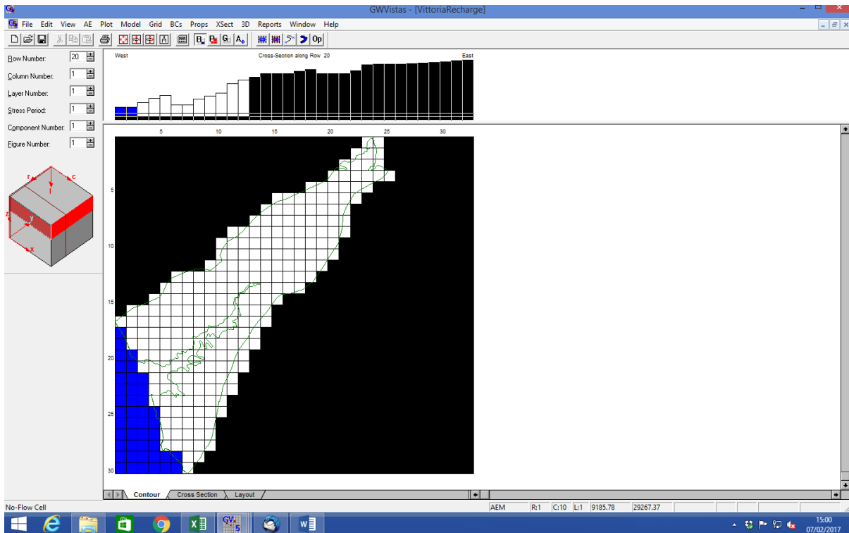
Figura 4.9 Condizione di carico idraulico costante pari a zero metri in corrispondenza delle celle che rappresentano la linea di costa e il mare e condizione di assenza di flusso nelle celle a destra e a sinistra della conoide alluvionale.
