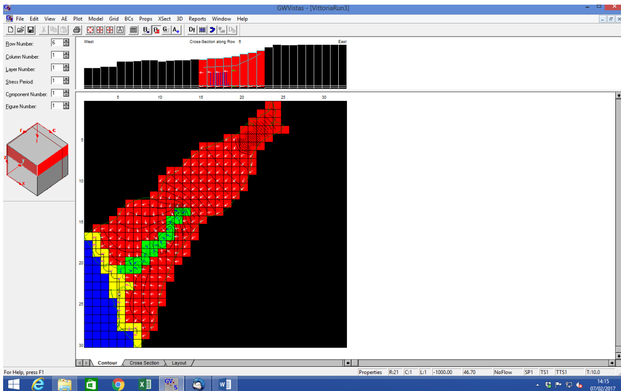
Figura 4.12 Curve iso-piezometriche e vettori di velocità simulate da MODFLOW per l'acquifero individuato nella piana di Vittoria.
