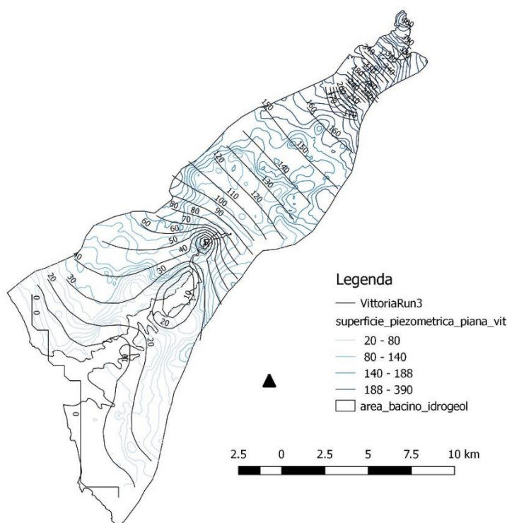
Figura 4.14 Curve iso-piezometriche osservate e simulate da MODFLOW per l'acquifero individuato nella piana di Vittoria.
