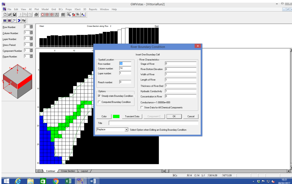
Figura 4.10 Inserimento delle caratteristiche del fiume ricadente nell'acquifero individuato nella Piana di Vittoria.
