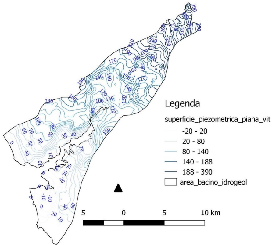
Figura 4.11 Linee iso-piezometriche elaborate a partire dalla banca dati di indagini di sottosuolo (ISPRA).
