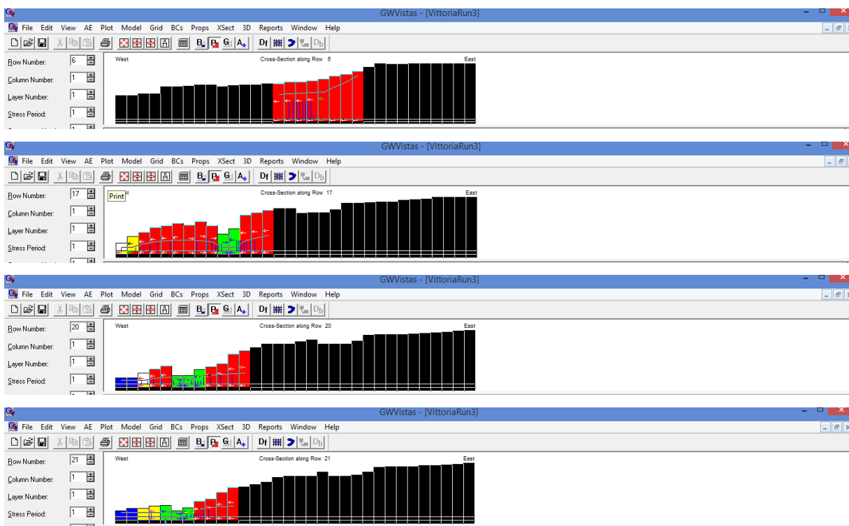
Figura 4.13 Sezioni significative dell'acquifero individuato nella piana di Vittoria e simulato con MODFLOW.
